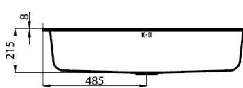
Серия Uragano Мод./Mod.1555/600
