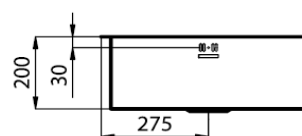
Серия Quadra под плот Мод./Mod.1215/890
